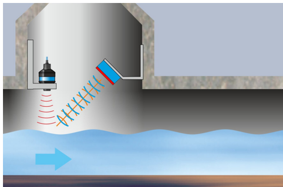
Impianto modulare di misura radar della portata con un livello di misurazione a ultrasuoni separato
