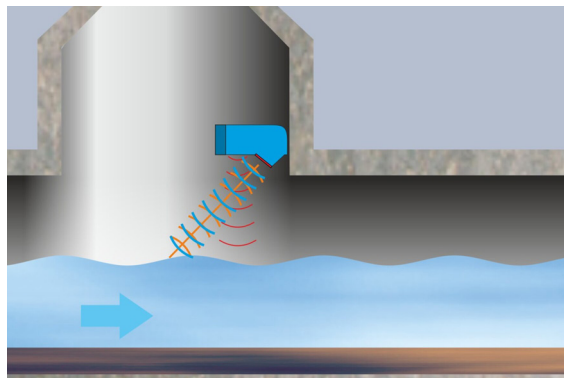
Impianto compatto di misura radar della portata con rilevamento del livello a ultrasuoni o radar in un unico alloggiamento
