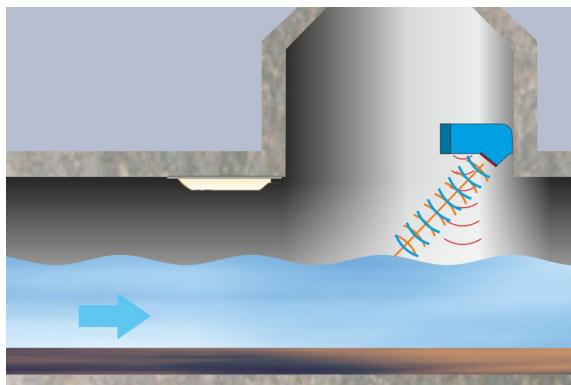
Condizioni normali: misurazione radar della portata con misurazione combinata del livello a ultrasuoni o radar in funzione. Il sensore di sovraccarico non è attivo a una portata di basso livello
