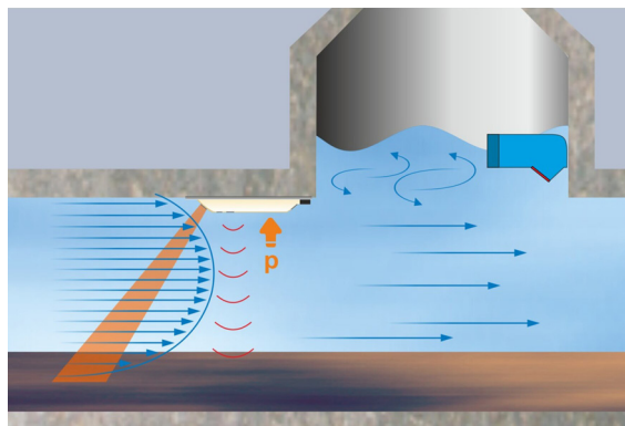
Condizioni di sovraccarico: la misurazione della portata a ultrasuoni rileva il profilo della portata con la misurazione combinata del livello idrostatico. Un'ulteriore misurazione del livello a ultrasuoni rileva i sedimenti a livello del suolo
